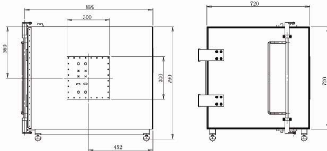
屏蔽箱内部尺寸为620X620X800。 表面喷白塑
